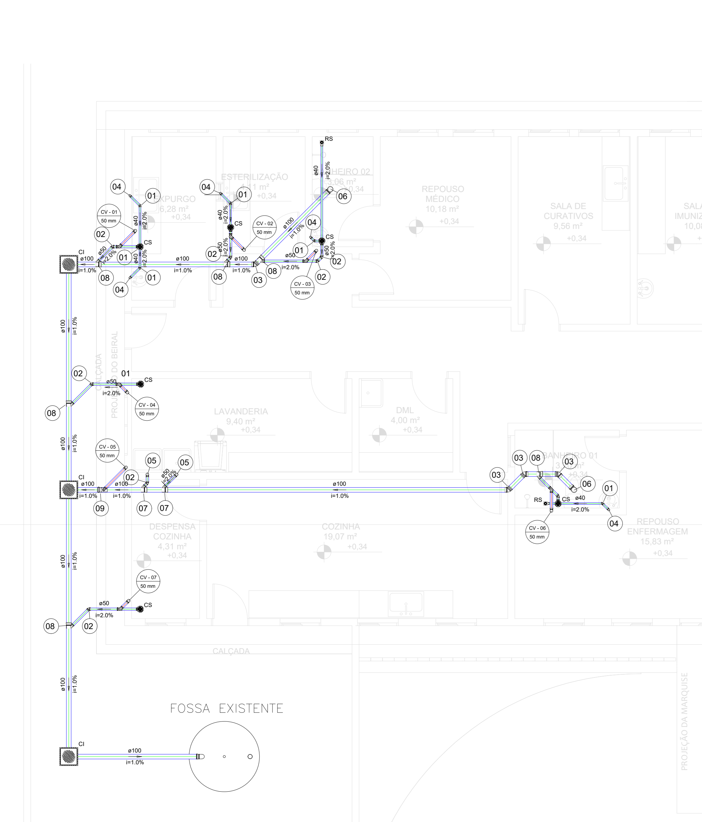
PLANTA BAIXA - ESGOTO ESCALA 1/50
