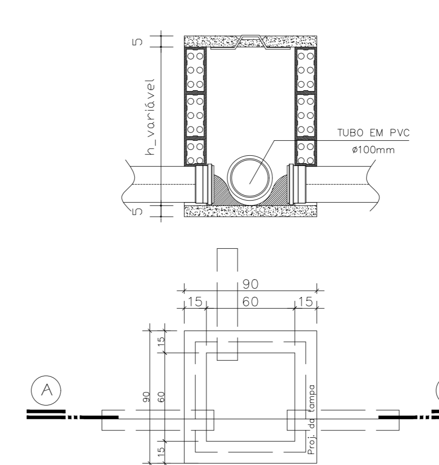
DETALHE CAIXA DE INSPEÇÃO SEM ESCALA
