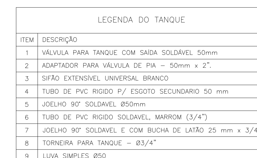
DETALHE TANQUE SEM ESCALA
