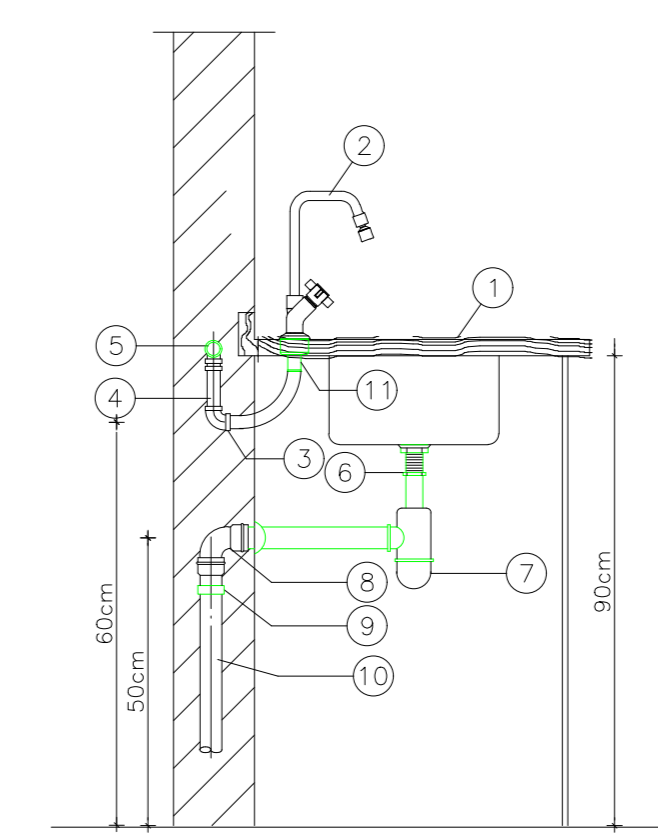
DETALHE DE INSTALAÇÃO DO LAVATÓRIO DE BANCADA SEM ESCALA
